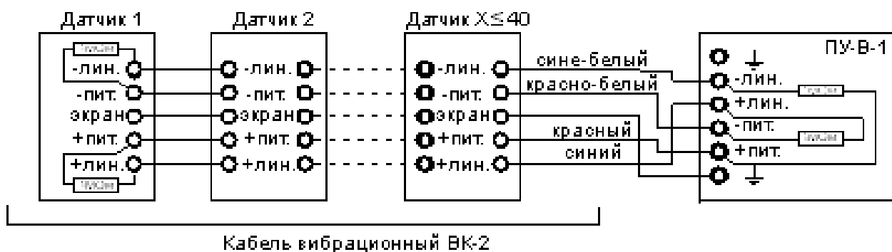
Рисунок 1 - Подключение кабеля к ПУ-В-1
